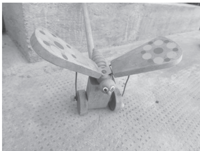
Az excentrikus kerékrögzítés miatt menet közben csattogó szárnyú „lepke”
